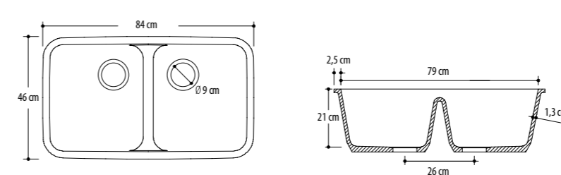
mod. DS 3116 84 x 46 x 21 cm
